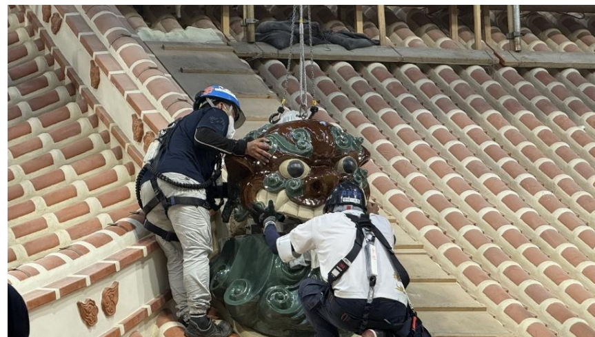
正殿鬼瓦設置状況 (R7 5/22)
