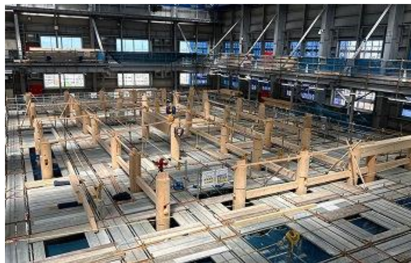
正殿木軸建方 下層柱建方中 3F 南側から北側望む (R5 9/28)
