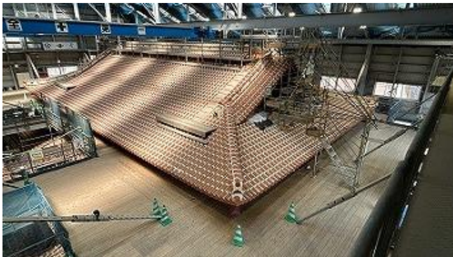
正殿 屋根工事 上層(久志間切弁柄上塗り施工中) 点検通路 南西側から北東側望む (R7 3/25)
