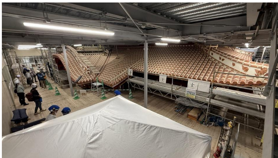
正殿 唐玻豊(からはふう)龍頭棟飾り設置中 2F 南側から北側望む (R7 5/22)
