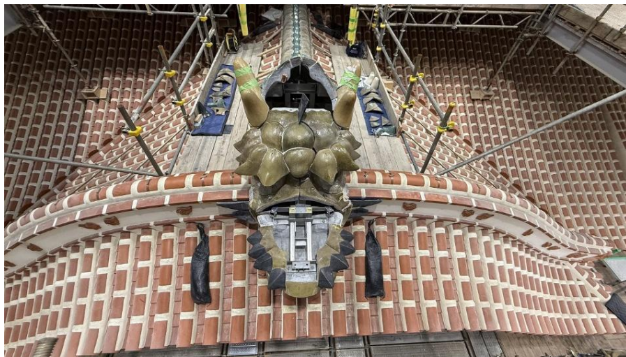
正殿 唐玻豊(からはふう)龍頭棟飾り設置中 3F 上側から望む (R7 5/22)
