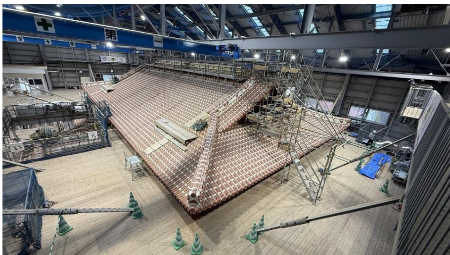
正殿 屋根工事 上層(龍頭棟飾り施工中) 点検通路 南西側から北東側望む (R7 5/22)
