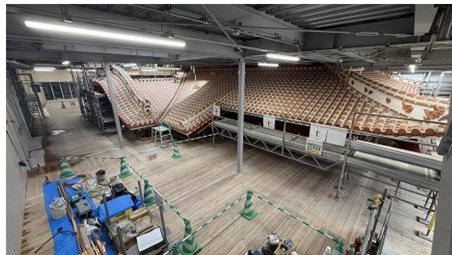
正殿 唐玻豊(からはふう)龍頭棟飾り設置中 2F 南側から北側望む (R7 6/25)
