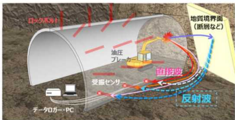
切羽前方の地山状況を探査
