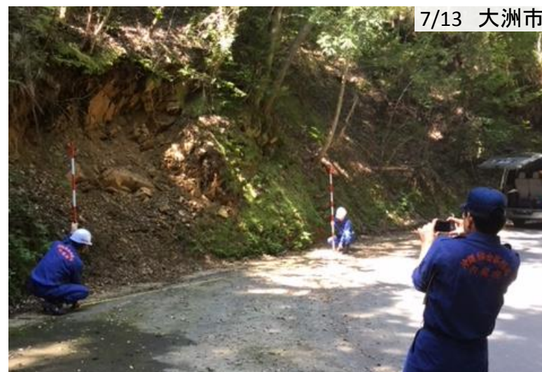
崩れた道路沿いの斜面を調査
