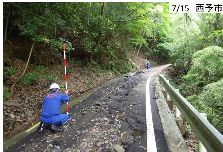
大雨によって大きな亀裂が発生した道路を調査
