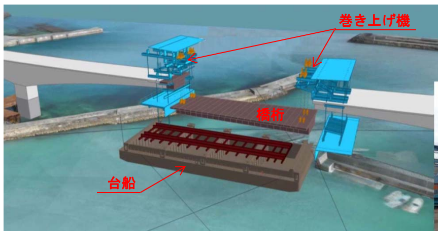
～一括架設のイメージ図～
