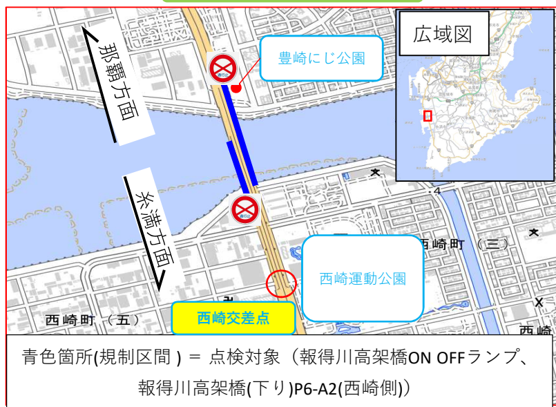
現場位置図
