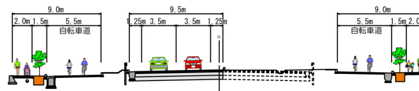
本線平面構造+歩道+自転車道(親志波平線～中央残波線)
