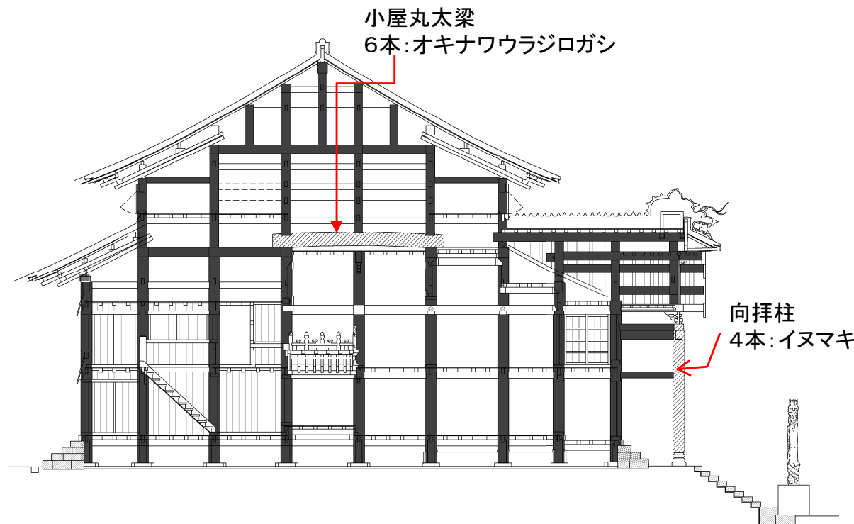
正殿 小屋丸太梁(オキナワウラジログシ)
