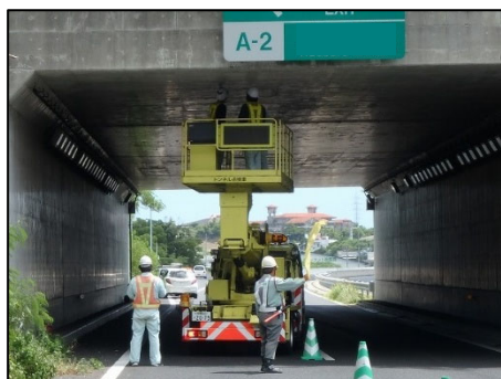
点検車による点検 （大型カルバート）
