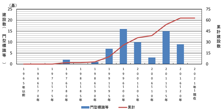
門型標識等供用数の推移
