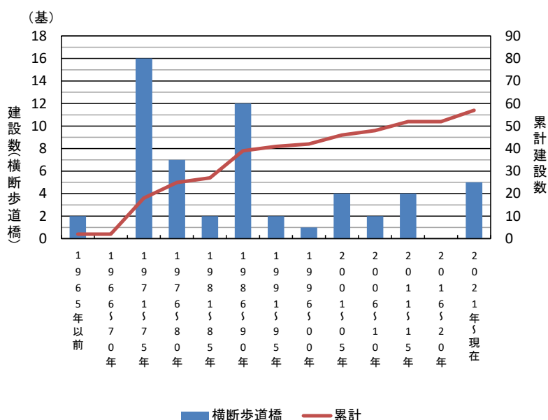
建設後50年以上の横断歩道橋数の推移
