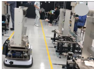
＜円研工程＞ S-CART ストッカー搬送
