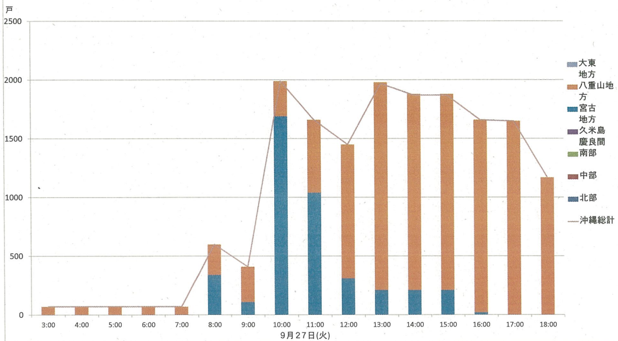
台風第17号による停電状況
