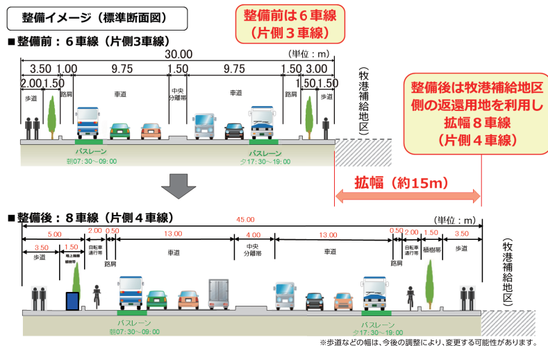
図-2 整備イメージ(標準断面図)
