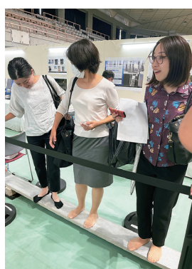
乗っても折れず、しなるコンクリート
