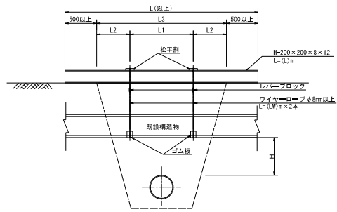
横断図
