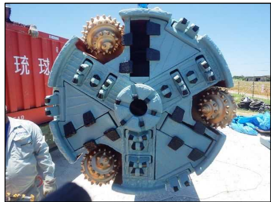
使用岩切削型ヘッド推進機
